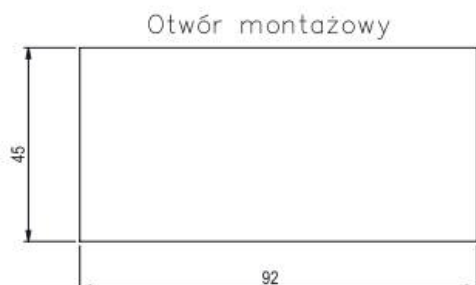
Wymiary CL600 w wersji panelowej
